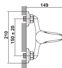
39360 Monomando para baño y ducha Equipo de ducha: ▪ Flexo de 150 cm ▪ Ducha de mano ▪ Soporte para mano de ducha
