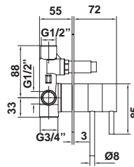
38892 Termostático empotrado para ducha (2 salidas)
