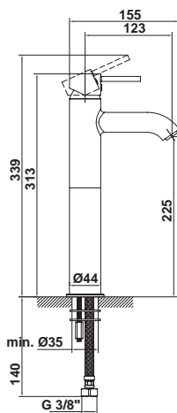
38923 Monomando de lavabo ECO con caño alto Cartucho ecológico Enlaces de alimentación flexible de 3/8" Aireador ecológico con limitador de caudal: ▪ Antivandálico ▪ Con filtro antipartículas integrado ▪ Protección contra la cal Instalación con válvula up-down*
