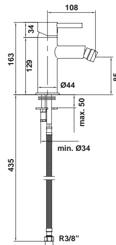
38887 Monomando de bidé Enlaces de alimentación flexible de 3/8" Instalación con válvula up-down*
