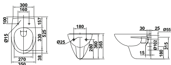
18172 Inodoro suspendido de 52,5 x 35 cm Salida horizontal. Posibilidad de instalación con soporte mural Ver p. 102-105
