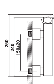
38774 Monomando de bidé Enlaces de alimentación flexible de 3/8" Instalación con válvula up-down.*
