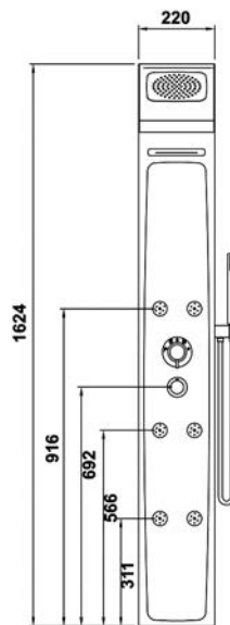
8019301 Columna SKY termostática de 162,4 x 22 cm
