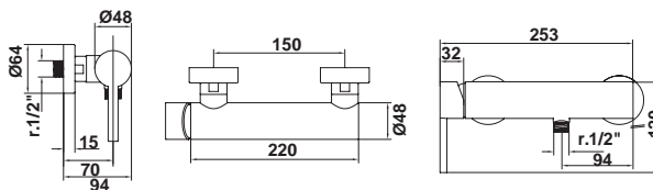
39318 Monomando para ducha Cartucho ecológico Equipo de ducha: ▪ Flexo de 175 cm ▪ Ducha de mano ▪ Soporte para ducha de mano
