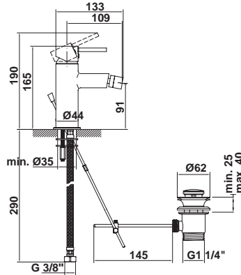
38925 Monomando de bidé ECO con desagüe automático Cartucho ecológico Enlaces de alimentación flexible de 3/8" Aireador ecológico con limitador de caudal
