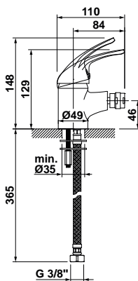
39357 Monomando de bidé Enlaces de alimentación flexible de 3/8"
