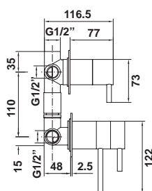
38895 Termostático empotrado para baño y ducha (3 salidas)
