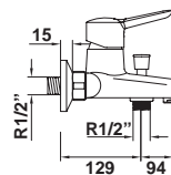
38836 Monomando para baño y ducha Equipo de ducha: • Flexo de 175 cm • Ducha de mano • Soporte para ducha de mano
