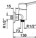
38835 Monomando para ducha Equipo de ducha: • Flexo de 175 cm • Ducha de mano • Soporte para ducha de mano
