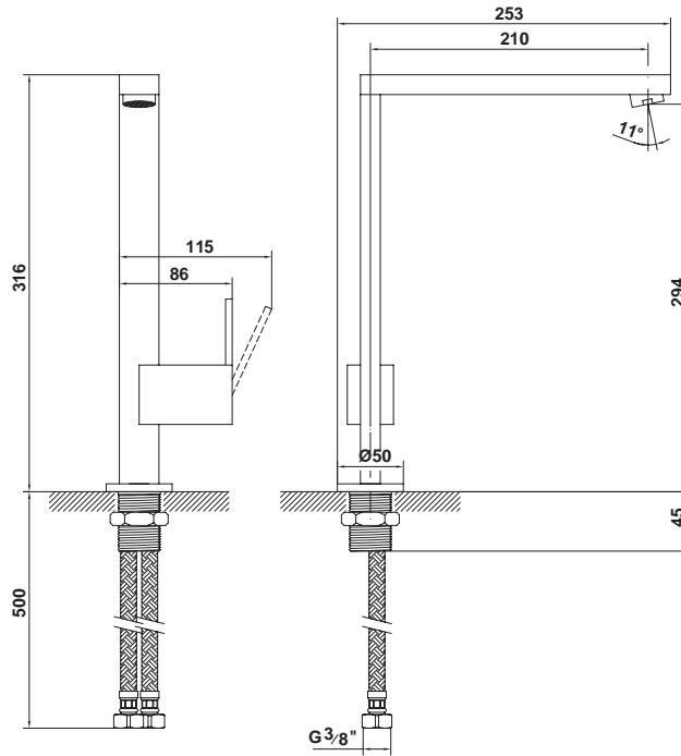
38782 Monomando de cocina. Caño giratorio Enlaces de alimentación flexible de 3/8"
