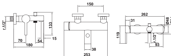
39317 Monomando para baño y ducha Cartucho ecológico Equipo de ducha: ▪ Flexo de 175 cm ▪ Ducha de mano ▪ Soporte para ducha de mano
