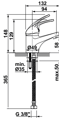
39355 Monomando de lavabo Enlaces de alimentación flexible de 3/8"
