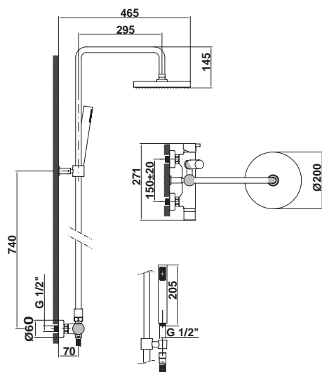
38928 Columna de ducha Equipo de ducha: ▪ Rociador de gran caudal de \text{Ø } 20 \text{ cm} ▪ Flexo de 175 cm ▪ Ducha de mano ▪ Soporte para ducha de mano integrado en la grifería
