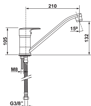
38993 Monomando de cocina Caño giratorio de 21 cm Enlaces de alimentación flexible de 3/8"
