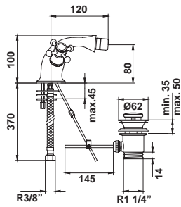
38971 Mezclador de bidé con desagüe automático Enlaces de alimentación flexible de 3/8" Montura cerámica 1/4 vuelta
