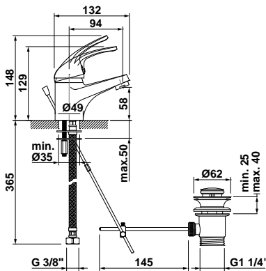
39356 Monomando de lavabo con desagüe automático Enlaces de alimentación flexible de 3/8"
