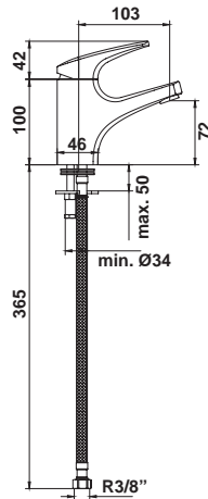
38931 Monomando de lavabo Cartucho ecológico Enlaces de alimentación flexible de 3/8" Instalación con válvula up-down*
