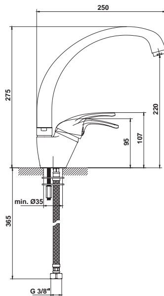
39361 Monomando de cocina Caño giratorio Enlaces de alimentación flexible de 3/8"
