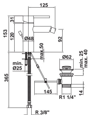
39314 Monomando de bidé con desagüe automático. Cartucho ecológico Enlaces de alimentación flexible de 3/8"
