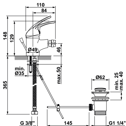
39358 Monomando de bidet con desagüe automático Enlaces de alimentación flexible de 3/8"
