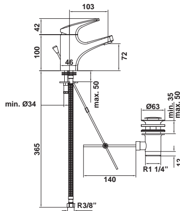
38930 Monomando de lavabo con desagüe automático Cartucho ecológico Enlaces de alimentación flexible de 3/8"
