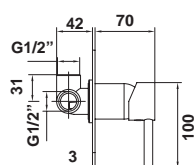
38889 Monomando empotrado para ducha
