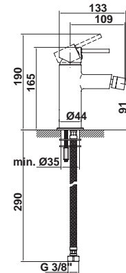
38924 Monomando de bidé ECO Cartucho ecológico Enlaces de alimentación flexible de 3/8" Aireador ecológico con limitador de caudal Instalación con válvula up-down.*
