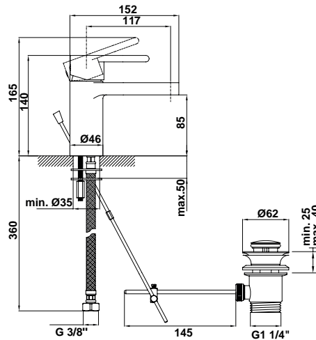
38960 Monomando de lavabo con desagüe automático Cartucho ecológico Enlaces de alimentación flexible de 3/8" Aireador antivandálico: • Con filtro antipartículas integrado • Protección contra la cal
