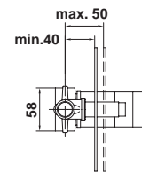
Thermostatique encastré pour douche (2 sorties)
