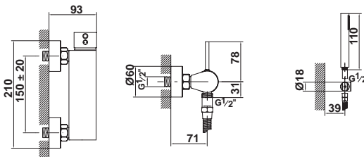
38926 Monomando para ducha ECO Incluye reductor de caudal Equipo de ducha: ▪ Flexo de 175 cm ▪ Ducha de mano ▪ Soporte para ducha de mano
