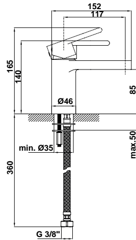
38961 Monomando de lavabo Cartucho ecológico Enlaces de alimentación flexible de 3/8" Aireador antivandálico: • Con filtro antipartículas integrado • Protección contra la cal Instalación con válvula up-down*
