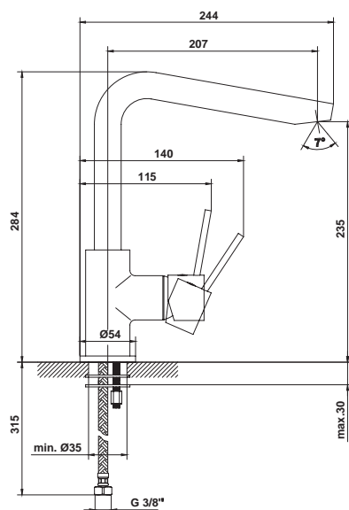
39335 Monomando de cocina Cartucho ecológico Caño giratorio Aireador orientable
